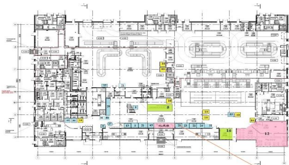
План 1-го этажа (из отв. 0.000). М 1:200
